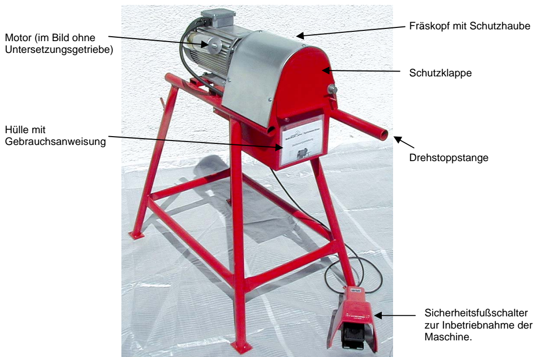
Abb. 5 Wacker Putz- und Fräsmaschine.
