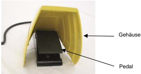
Abb. 4 Sicherheitsfußschalter.
